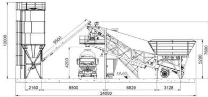
A-A SECTION
